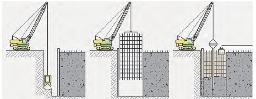
Figura 8: proceso de ejecución de muro pantalla de hormigón armado in situ con lodos.
