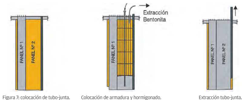
Figura 7: colocación de tubo-junta.
