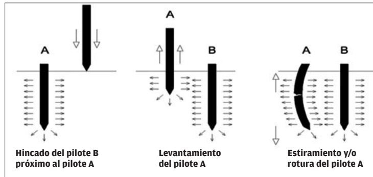
Figura 9: lesiones o daños en pilote por hincado próximo de otro pilote.
