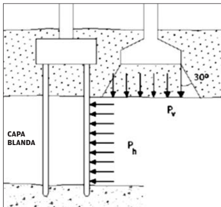
Figura 6: empujes horizontales producidos por cargas superficiales.
