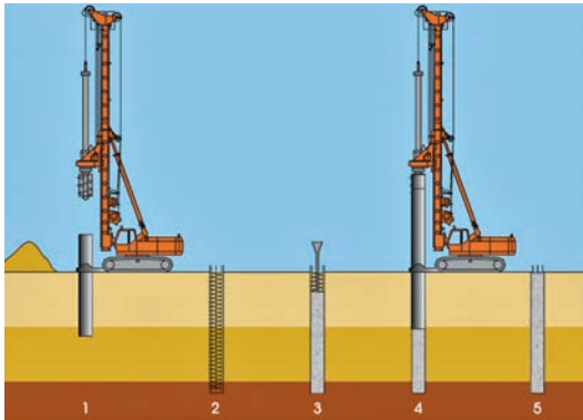
Figuras 1 y 2: ejecución de pilotes.
