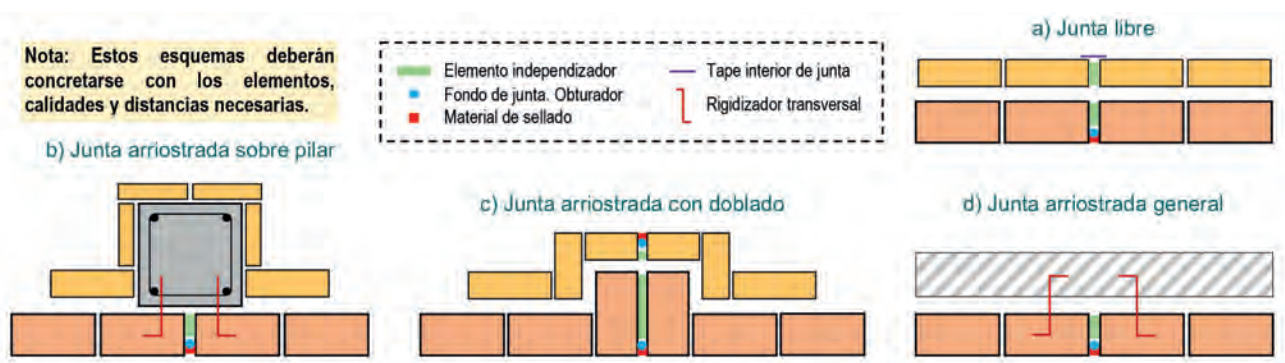
Figura 7: esquema de los distintos formatos de juntas de dilatación de fachada. Ejemplo para cerramientos de fábrica de ladrillo.
